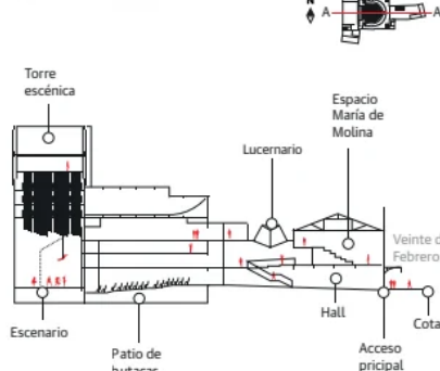
Sección longitudinal AA'
